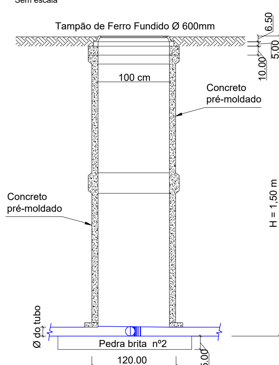
Detalhamento do poço de visita (PV): Sem escala
