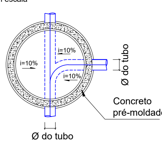
Detalhe do fundo (PV): Sem escala
