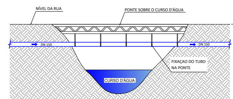
CROQUI DE DETALHAMENTO TUBAÇÃO SOBRE O CURSO D'ÁGUA SERÁ FIXADA NA PONTE Escala Sem Escala
