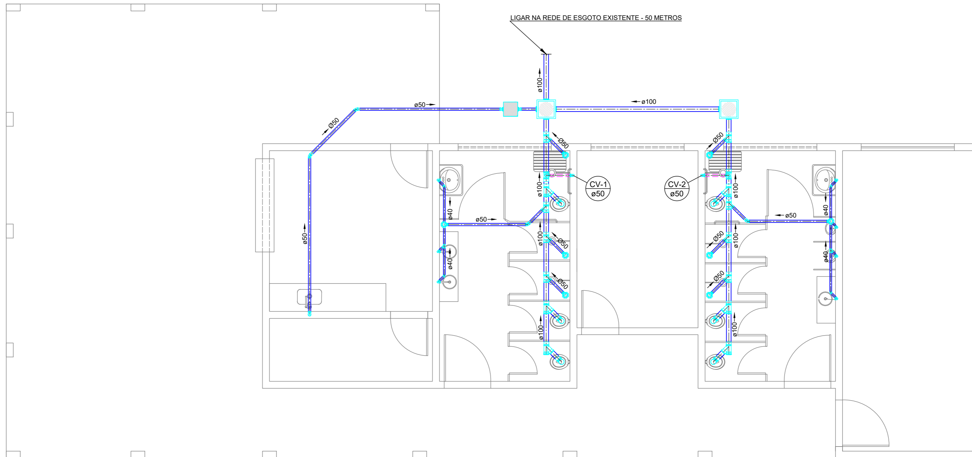
PLANTA TÉRREA REDE DE ESGOTO ESC.: 1/50
